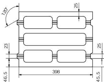
! technický náčrtek - dělitelná !
