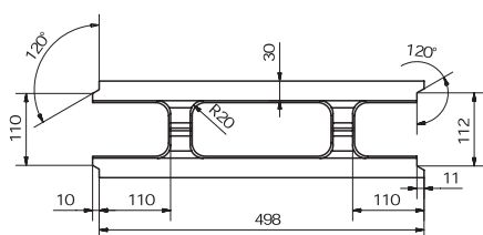
I technický náčrtek - dělitelná I
