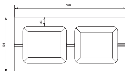
! technický náčrtek - dělitelná !
